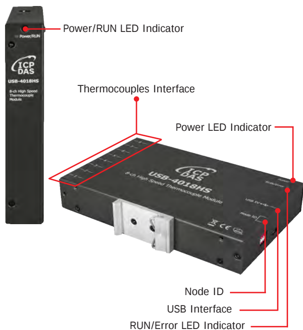
USB-4018HS
