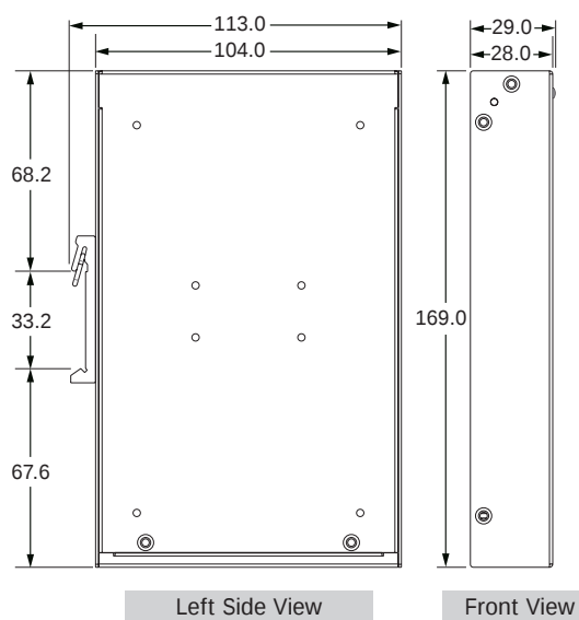
USB-4018HS
