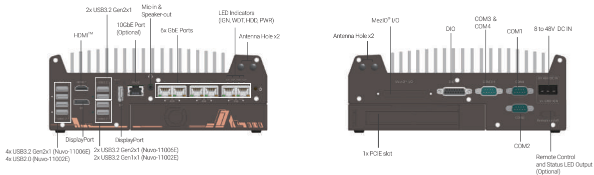
Nuvo-11000E
